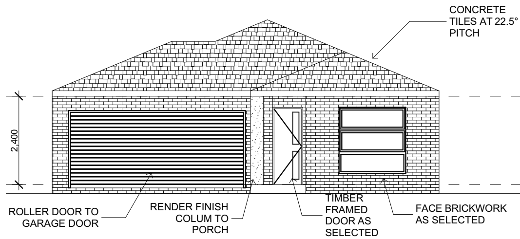
ELEVATION A
